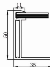
A-A
